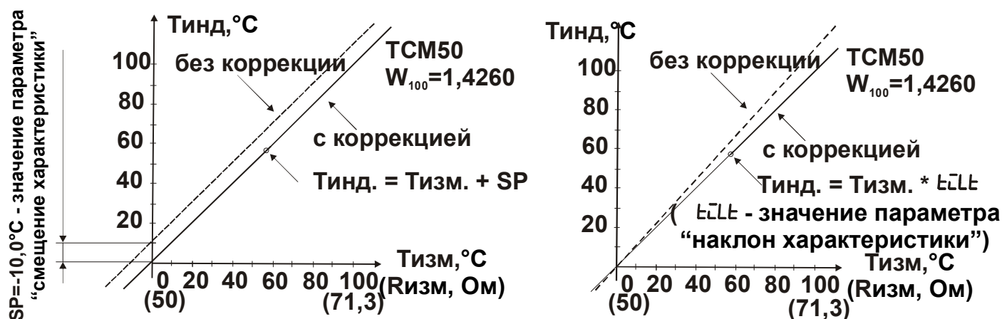
Рисунок 3.13 - Влияние параметров “Смещение характеристики” и “Наклон характеристики” на характеристику преобразования
